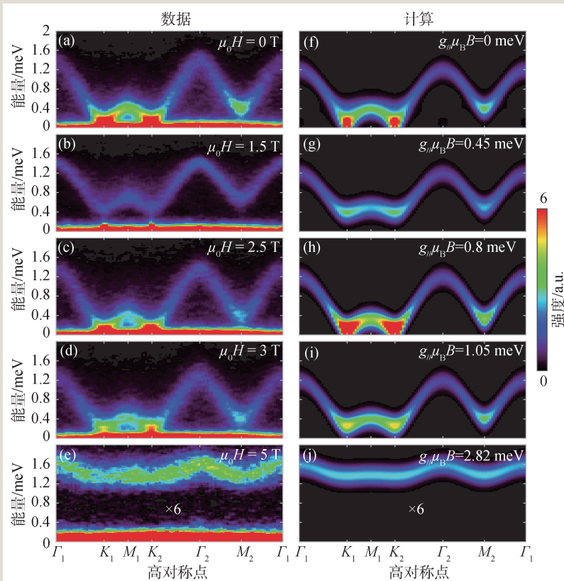
图7 \text{TmMgGaO}_4 的磁激发色散关系 [61] (a)–(e)沿着图5(b)所示高对称方向的中子散射强度随外场的变化; (f)–(j)横场伊辛模型的线性自旋波计算结果
