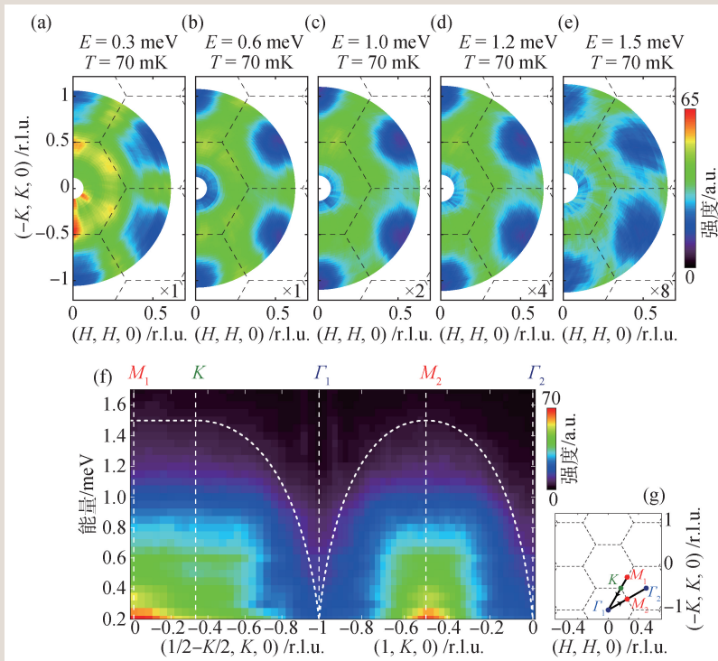
图2 YbMgGaO 4 中的自旋子激发 [37] (a)–(e) 自旋子激发在 HK0 面内的强度分布；(f) 自旋子激发沿着 (g) 中所示高对称方向的色散关系；(g) 倒空间示意图
