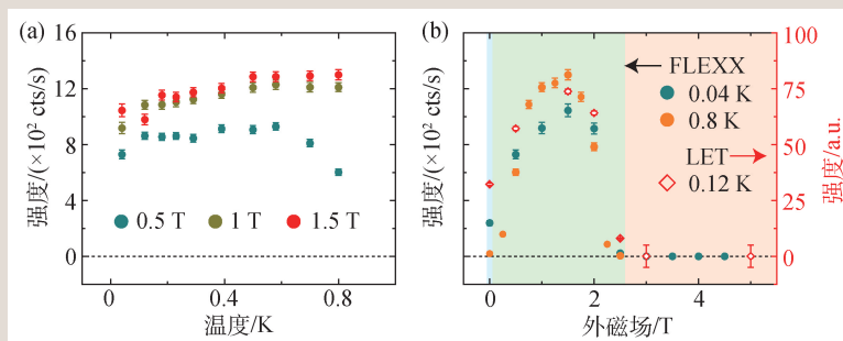
图8 外场下 \text{TmMgGaO}_4 的 K 点磁性布拉格峰强度随外场和温度的变化关系 [61] (a)不同外场下磁性布拉格峰随温度的变化关系; (b)不同温度下布拉格峰强度随磁场的变化关系,数据采自FLEXX和LET谱仪
