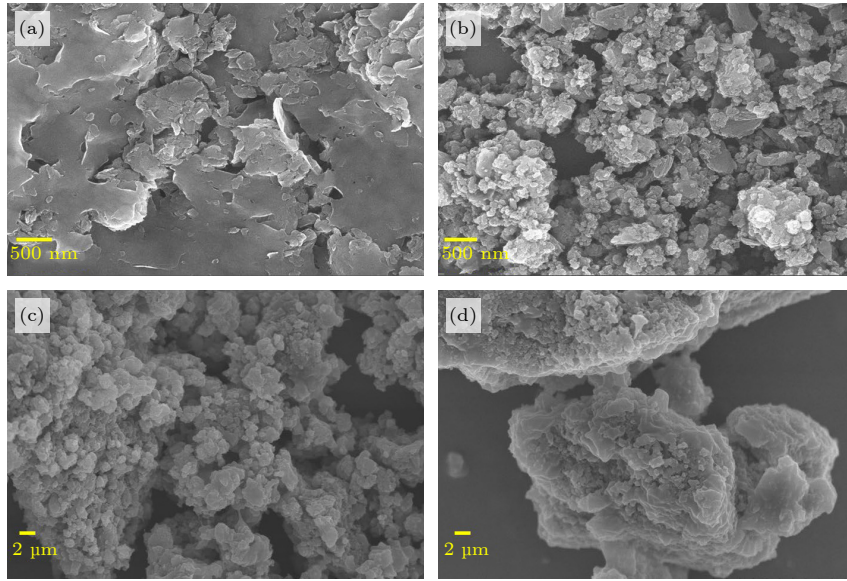
图 2 (a)–(d) 分别为 Co-BDC, Fe-BDC, \text{Co}_{0.1}\text{Fe}_{0.9} -BDC 和 \text{Co}_{0.5}\text{Fe}_{0.5} -BDC 的 SEM 图像
